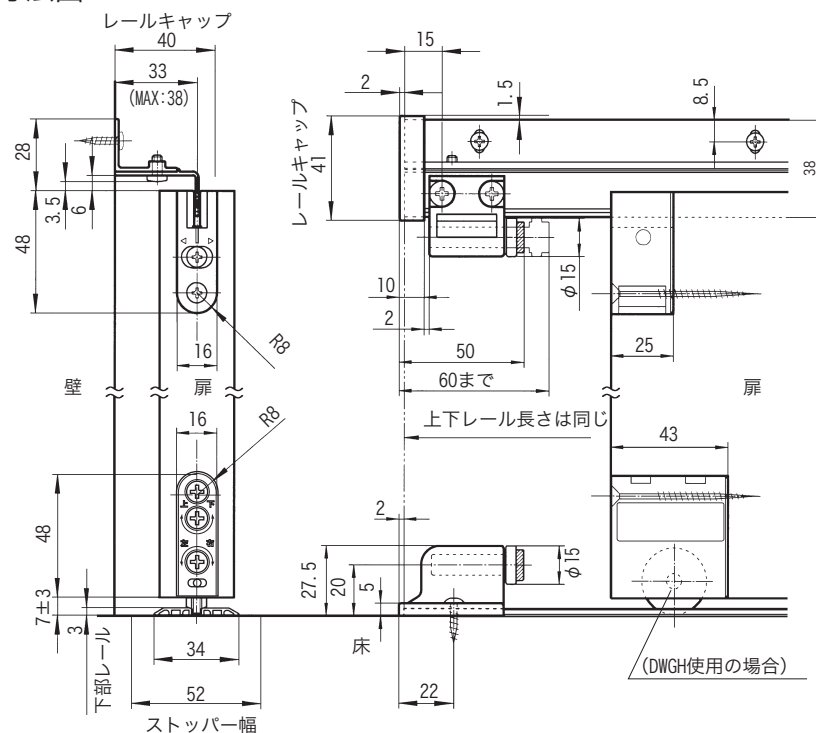
寸法図
